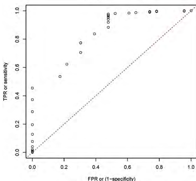
ROC Curve (AUC = 0.867)
